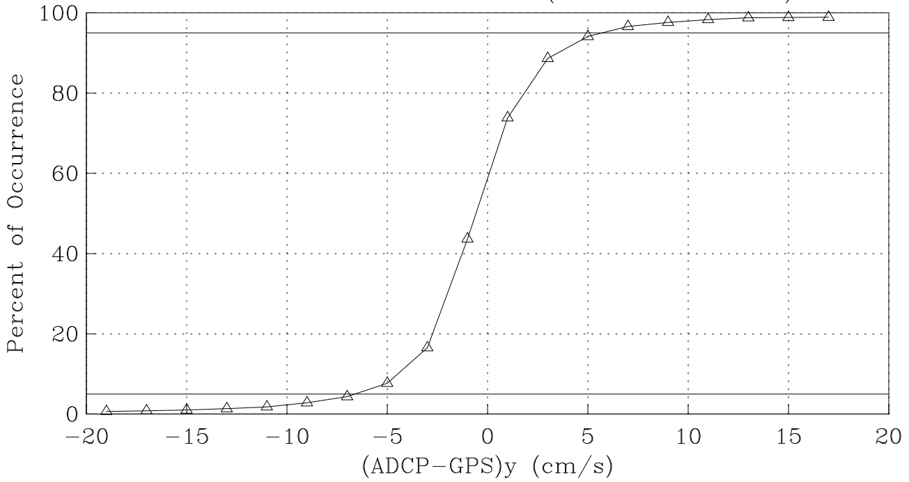
CATS-2003 ADCP Calibration (10-18-2004 amue)
