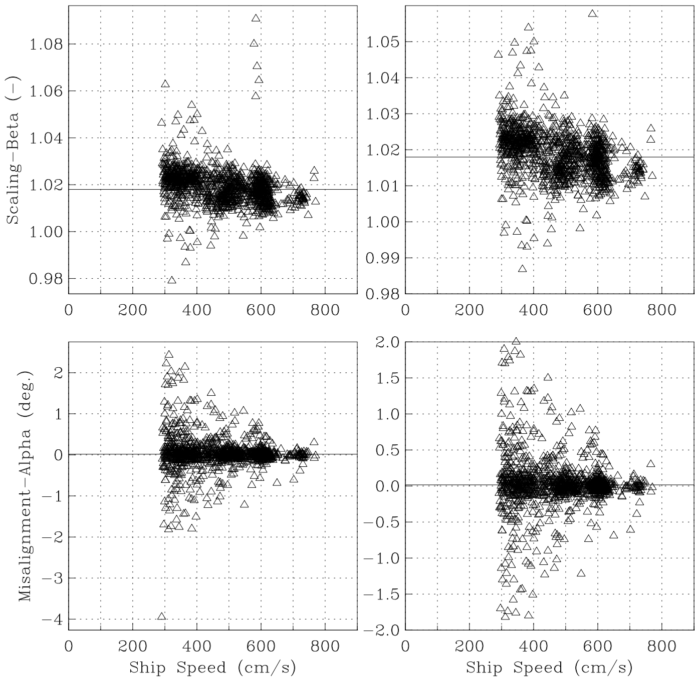
CATS-2003 ADCP Calibration (10-18-2004 amue)
